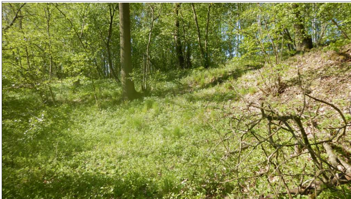
Morfologia koluwium w górnej części osuwiska
