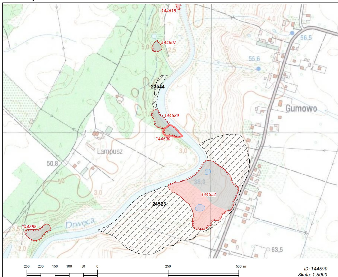
Szkic osuwiska nr 144590
