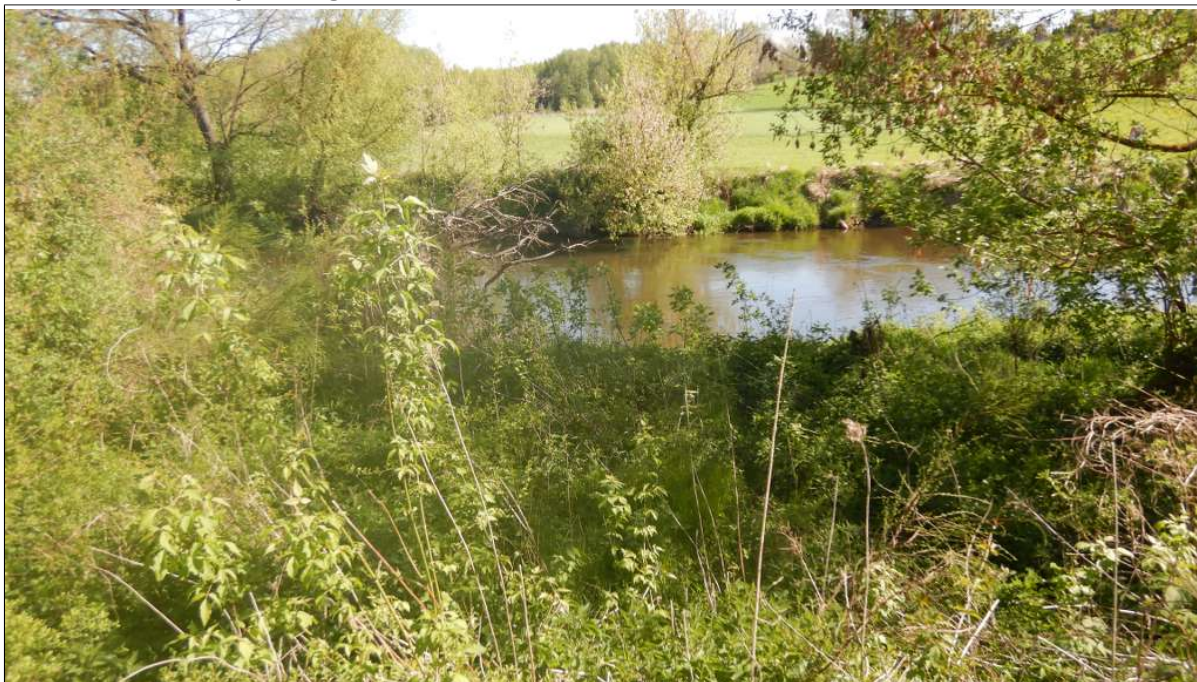
Koluwium w dolnej części osuwiska
