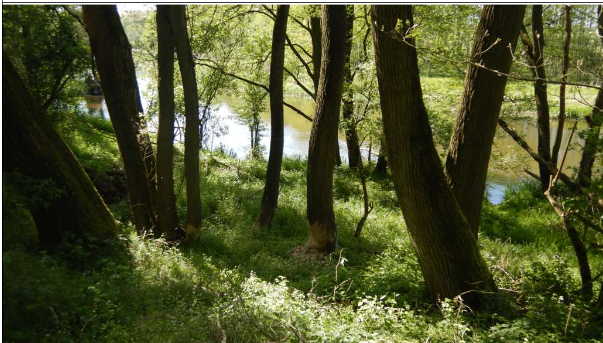
Koluwium w postaci progu wypchnięte w stronę koryta Drwęc
