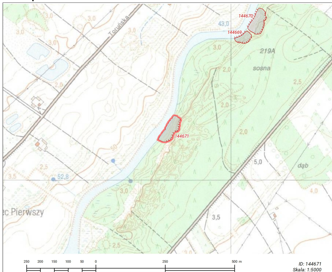
Szkic osuwiska nr 144671
